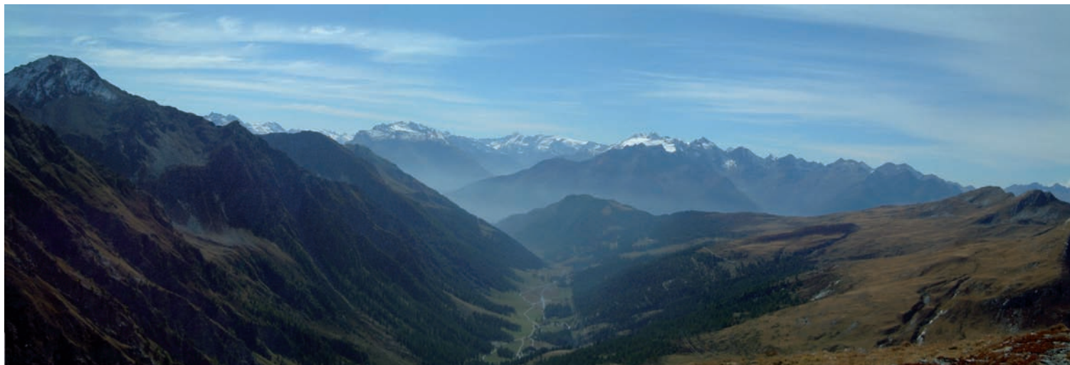
Fig. 15.7 - Panorama del vallone di Vertosan. Il fianco sinistro, più acclive, è impostato entro le unità di basamento (gneiss e micascisti) della Falda del Gran San Bernardo, mentre quello destro, più dolce, è modellato nelle unità di copertura carbonifere (scisti e filladi)
