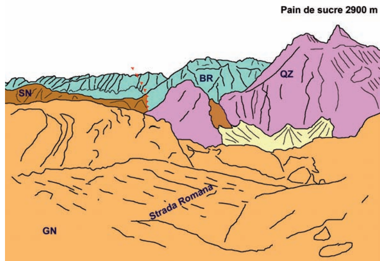
Fig. 15.3 - schizzo geologico dal Colle del Gran San Bernardo verso ovest. In primo piano le unità di basamento GN (gneiss polimetamorfici), in secondo piano le unità di copertura SN (scisti neri) e QZ (quartziti) della Falda del Gran San Bernardo. Più in lontananza il sovrascorrimento delle falde penninche esterne e l'Unità delle Breccie di Tarantasia (BR)
