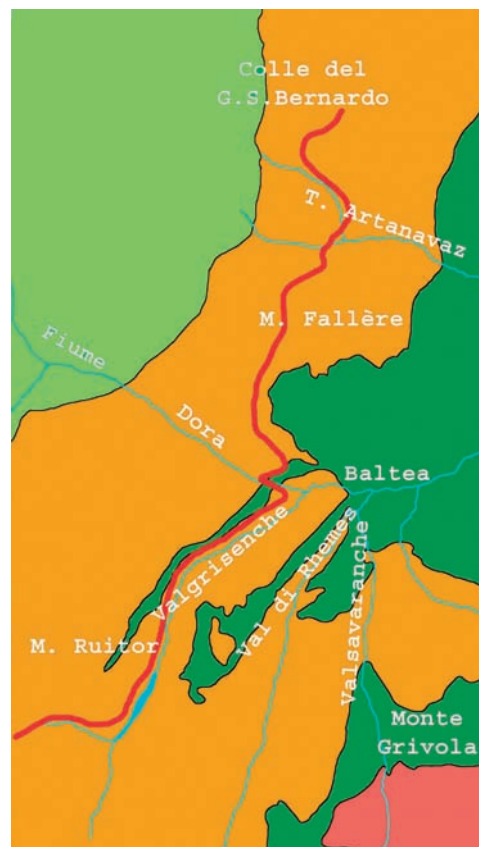
Fig. 15.2 - schema geologico semplificato dell'area: in marrone la falda del Gran San Bernardo, in verde scuro il Complesso dei Calcescisti con Pietre Verdi, in rosso l'itinerario
