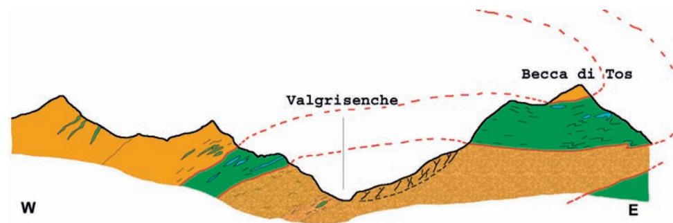
Fig. 15.15 - profilo geologico attraverso la media Valgrisenche, che illustra i ripetuti fenomeni di sovrascorrimento tra le rocce della falda del Gran San Bernardo (in marrone) e quelle dei Calcescisti con Pietre Verdi (in verde scuro), con la piega retroflessa della Becca di Tos
